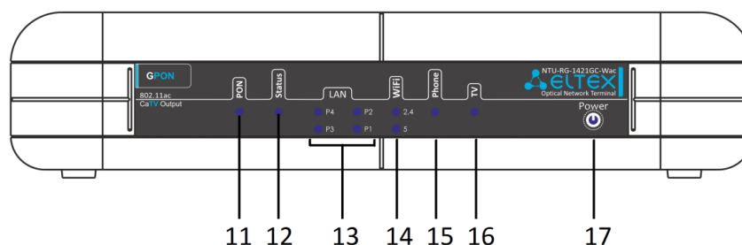
Рисунок 6 – Внешний вид передней панели NTU-RG-1421GC-Wac
